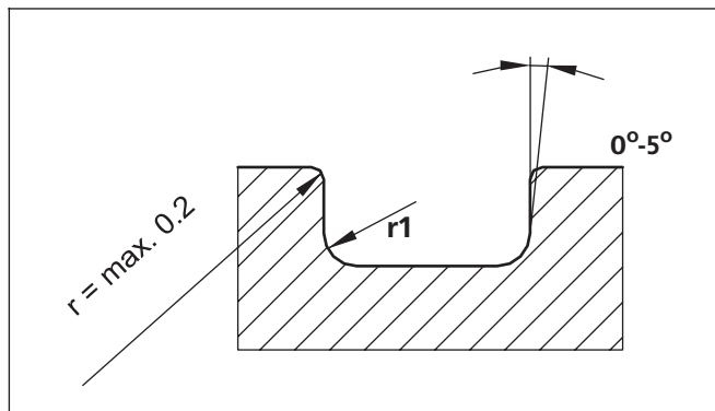
图24 沟槽尺寸
