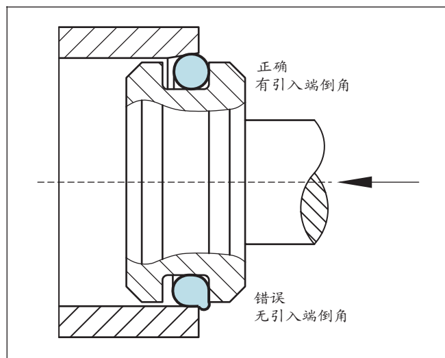
图12 装有O形密封圈的活塞的安装
